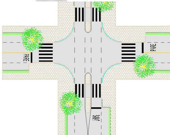
Figura 2 - Travessias com Alargamento de Calçadas
