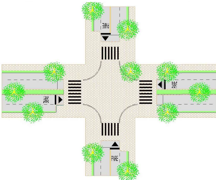
Figura 4 – Platô: Elevação em todo o Cruzamento
